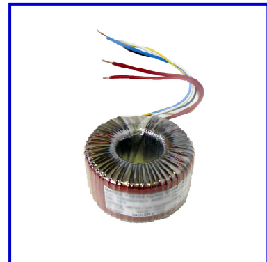
Ringkern-Transformator Schutzart IP00, T40/E mit losen Enden
